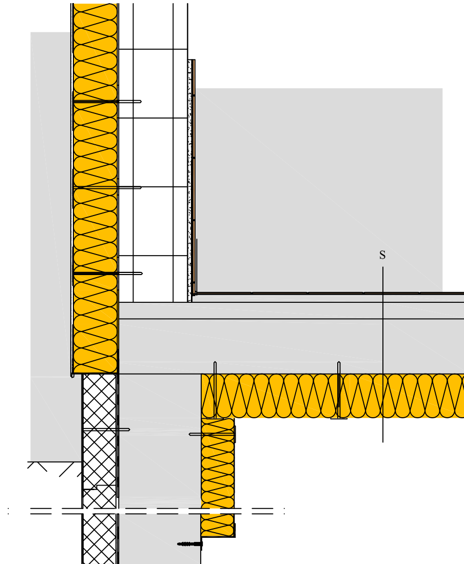
Secțiunea S - grosimi în cm
